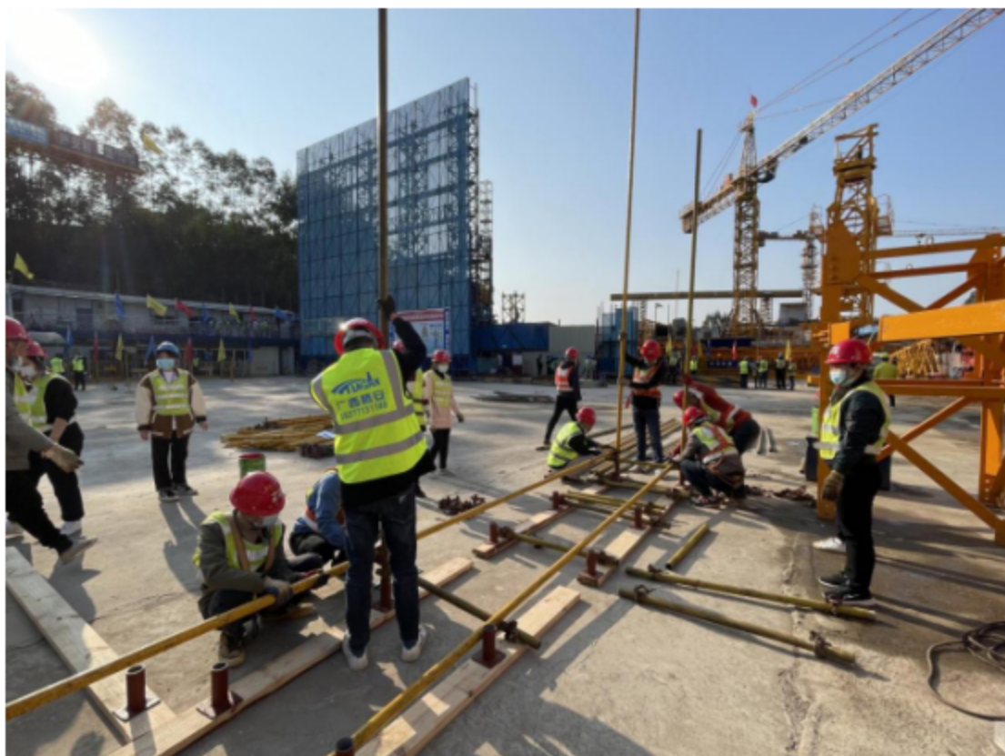
学员在进行脚手架搭设实操
